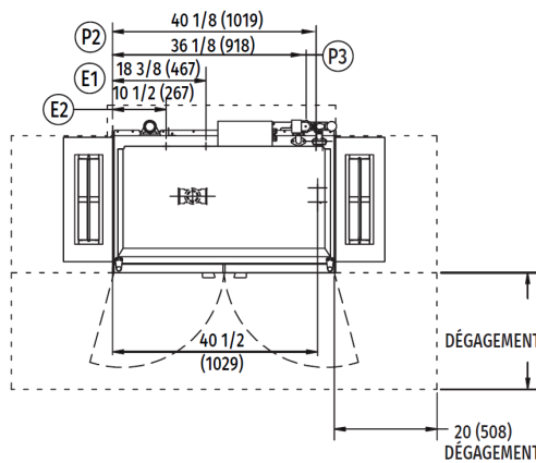
Vue en plan – G/D
