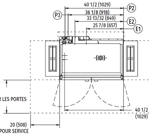
Vue en plan – D/G
