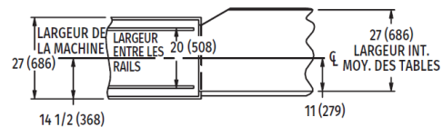
Agencement des tables et rails proposé
