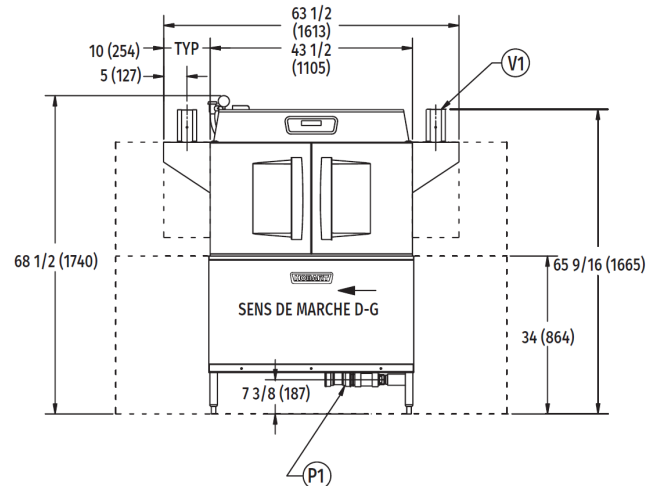
Vue de face D-G
