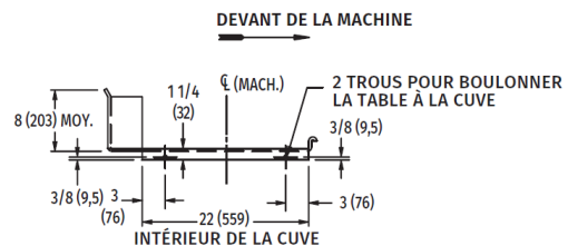
Vue indiquant la position des trous dans le bord recourbé de la table
