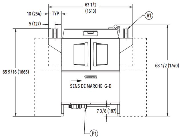
Vue de face G-D
